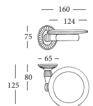
7006 PORTA-BICCHIERE GLASS HOLDER
