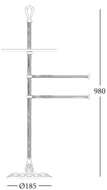
7216 PIANTANA ATTREZZATA EQUIPPED COLUMN
