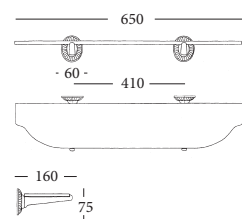
7011 MENSOLA SHELF
