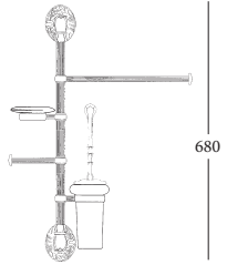
7217 COLONNA A MURO ATTREZZATA EQUIPPED WALL BAR
