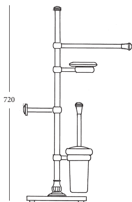
7015 PIANTANA ATTREZZATA EQUIPPED COLUMN
