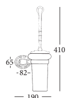
7209 PORTA-SCOPINO DA TERRA TOILET BRUSH HOLDER
