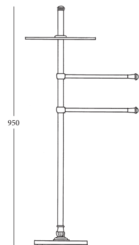
7016 PIANTANA ATTREZZATA EQUIPPED COLUMN
