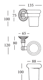
7006 PORTA-BICCHIERE GLASS HOLDER
