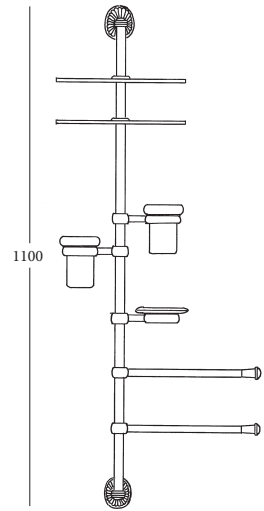
7018 COLONNA A MURO ATTREZZATA EQUIPPED WALL BAR
