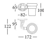
7206 PORTA-BICCHIERE GLASS HOLDER
