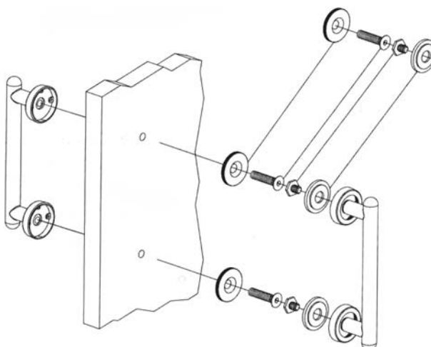
sistema di fissaggio di una coppia di maniglioni su porta legno (maniglioni con rosette art.102-103). accessori da ordinare separatamente (rif. listino prezzi art.118mn) / system for fixing a pair of pull handles on a wooden door (pull handles on rose art.102-103). fixing accessories to order separately (ref. price list art.118mn)
