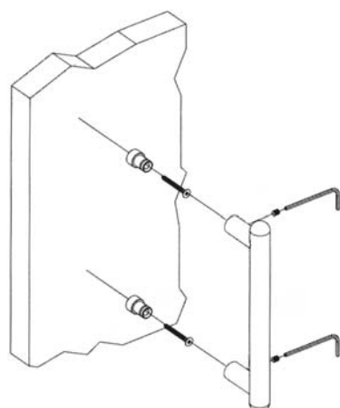
sistema di fissaggio singolo maniglione su porta in legno / fixing system for a single pull handle on a wooden door
