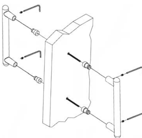
sistema di fissaggio di una coppia di maniglioni su porta legno / system for fixing a pair of pull handles on a wooden door
