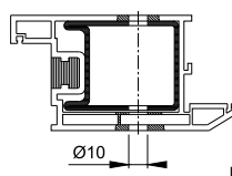
Kunststoff-Profil
