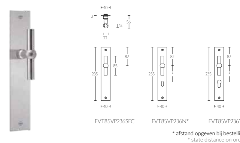
FVT85VP236 massieve knop vast op schild | solid knob fixed on plate
