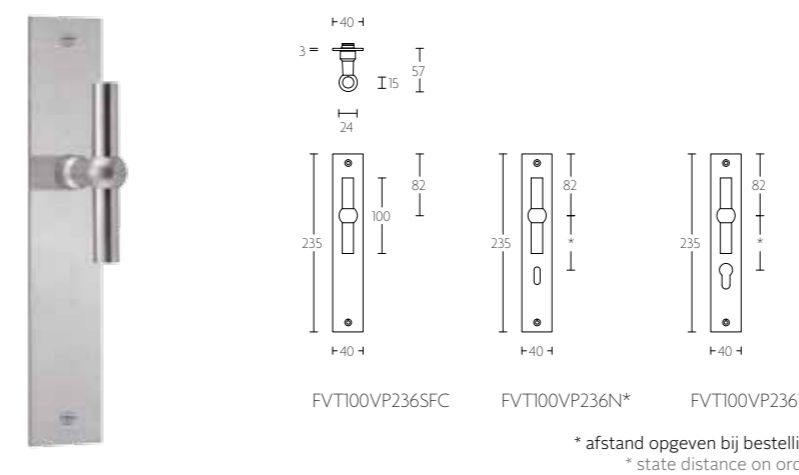
FVT100VP236 massieve knop vast op schild | solid knob fixed on plate
