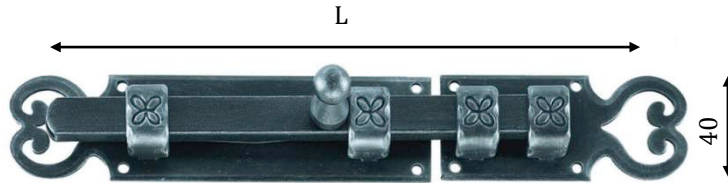
Art. 2118/ Catenaccio Traverso Horizontal Bolt
