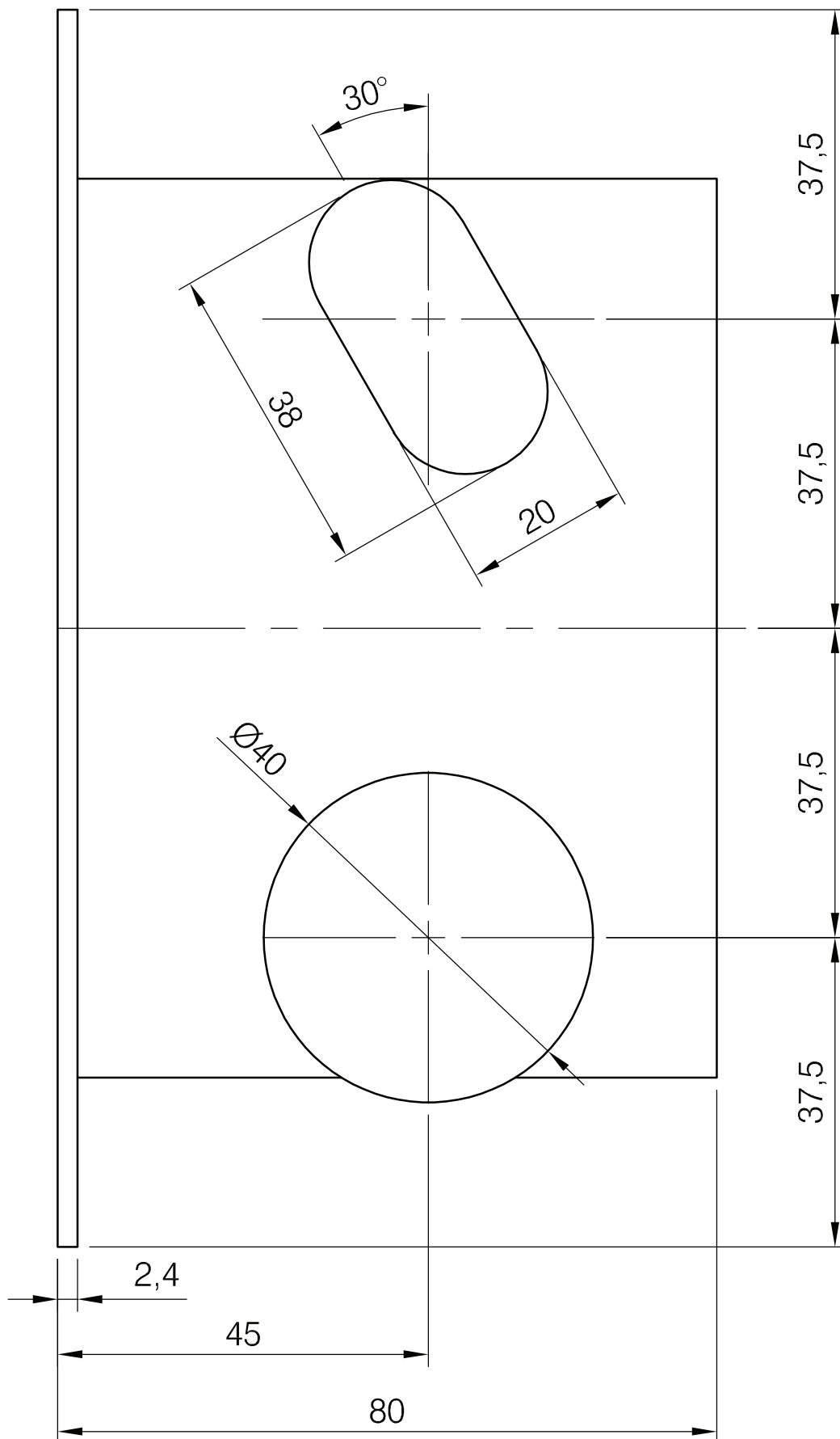
Lukukorpus / Lock case: Abloy 2014
