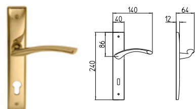
350 MANIGLIA PER PORTA CON PIASTRA door-handle on back plate
