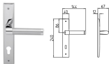
360 MANIGLIA PER PORTA CON PIASTRA door-handle on back plate
