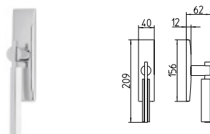
3182/M CREMONESE IMPUGNATURA MANIGLIA window lever-handle
