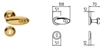
1111 MANIGLIA PER PORTA CON ROSETTA door-handle on rose
