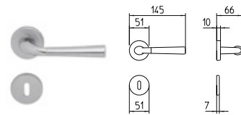
S101 MANIGLIA PER PORTA CON ROSETTA door-handle on rose
