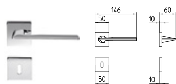
1461 MANIGLIA PER PORTA CON ROSETTA door-handle on rose
