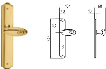
1110 MANIGLIA PER PORTA CON PIASTRA door-handle on back plate
