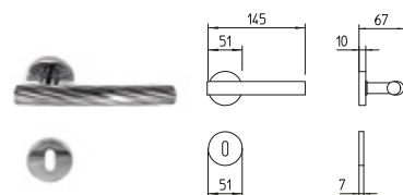
1731 MANIGLIA PER PORTA CON ROSETTA door-handle on rose
