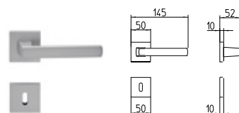
1291 MANIGLIA PER PORTA CON ROSETTA door-handle on rose
