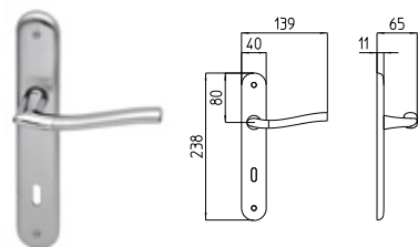
1180 MANIGLIA PER PORTA CON PIASTRA door-handle on back plate
