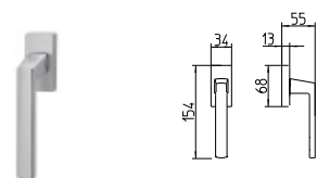
1292/DK MARTELLINA DK drehkipp system
