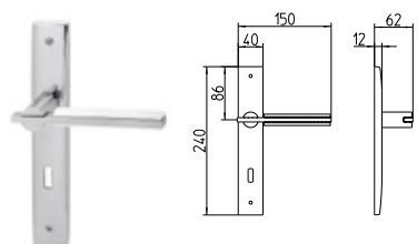
3180 MANIGLIA PER PORTA CON PIASTRA door-handle on back plate
