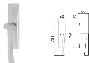
1072/M CREMONESE IMPUGNATURA MANIGLIA window lever-handle
