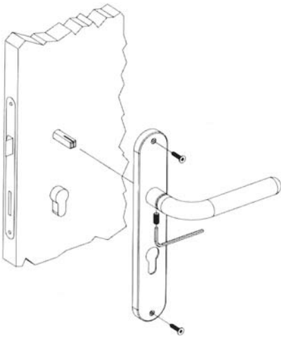
sistema di montaggio per maniglia con placca / fixing system for door handle on plate
