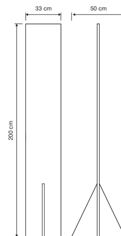
espositore da pavimento bifacciale floor display 061 AC
